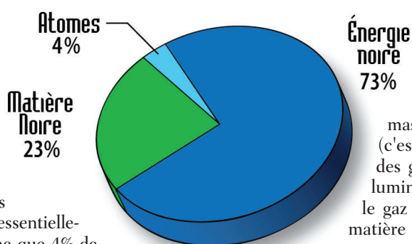
1. Le contenu en masse-énergie de l'Univers. © NASA
