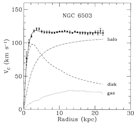
2. Courbe de rotation de galaxie.
