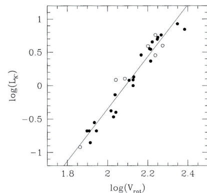
3. La Loi de Tully-Fisher.
